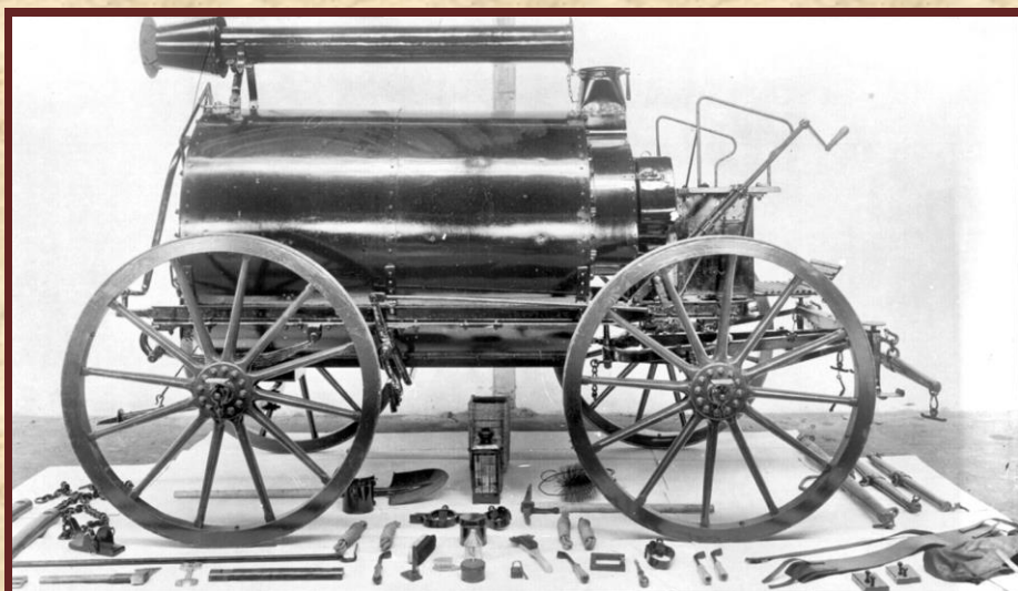
polní pekárna
