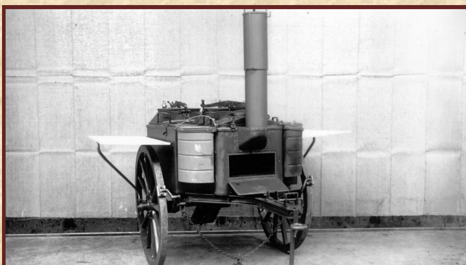
polní kuchyně
